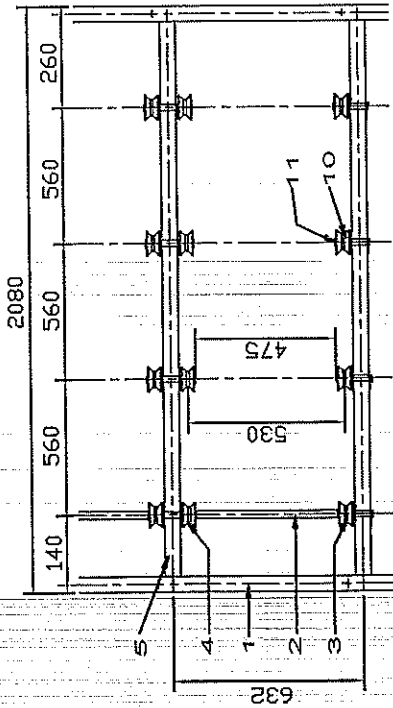
TOP ELEVATION
