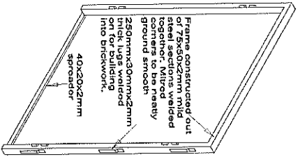
DOUBLE DOOR FRAME DETAILS
